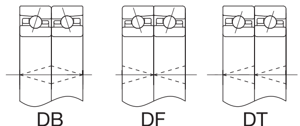
万能组合轴承的组合方式
